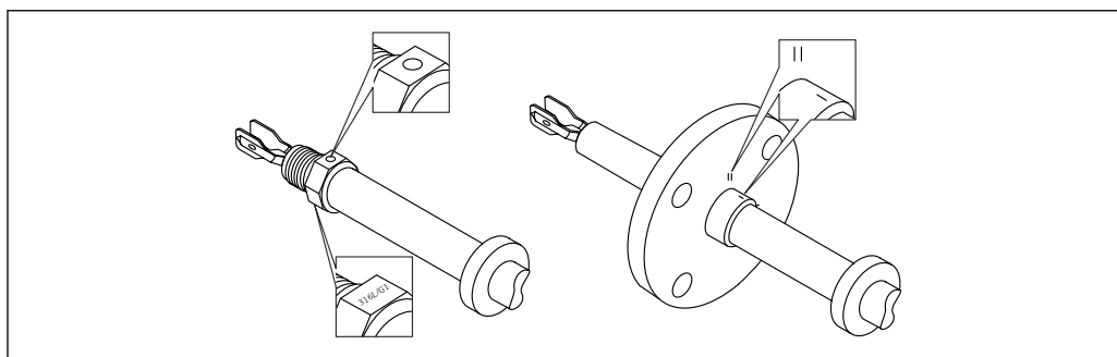
图 11 音叉安装位置标记
