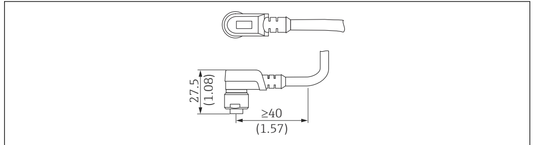
图 47 M12 插头, IP67 防护等级。测量单位 mm (in)
