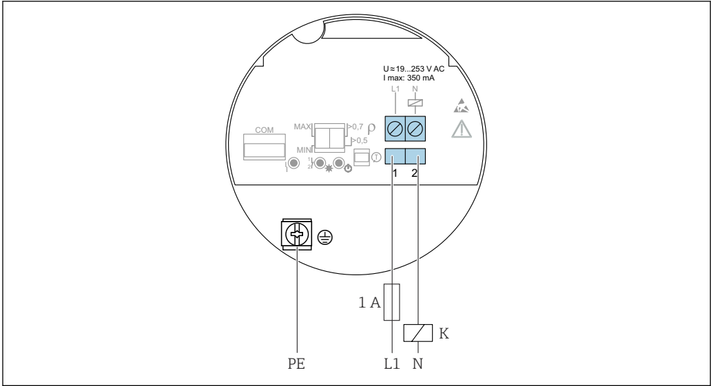
16 FEL61 电子插件：两线制连接，交流 AC 型
