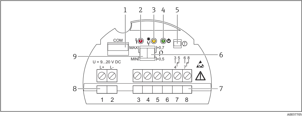
图 32 实例：电子插件 FEL64DC 1 通信接口，用于连接附加模块（LED 指示灯、蓝牙模块） 2 红色 LED 指示灯：警告或报警 3 黄色 LED 指示灯：继电器的开关状态 4 绿色 LED 指示灯：工作状态（设备开启） 5 测试按钮，用于执行功能测试 6 DIP 开关，密度设定值为 0.7 或 0.5 7 继电器触点接线端子（3...8） 8 电源接线端子（1...2） 9 DIP 开关，高限（MAX）/低限（MIN）检测设置
