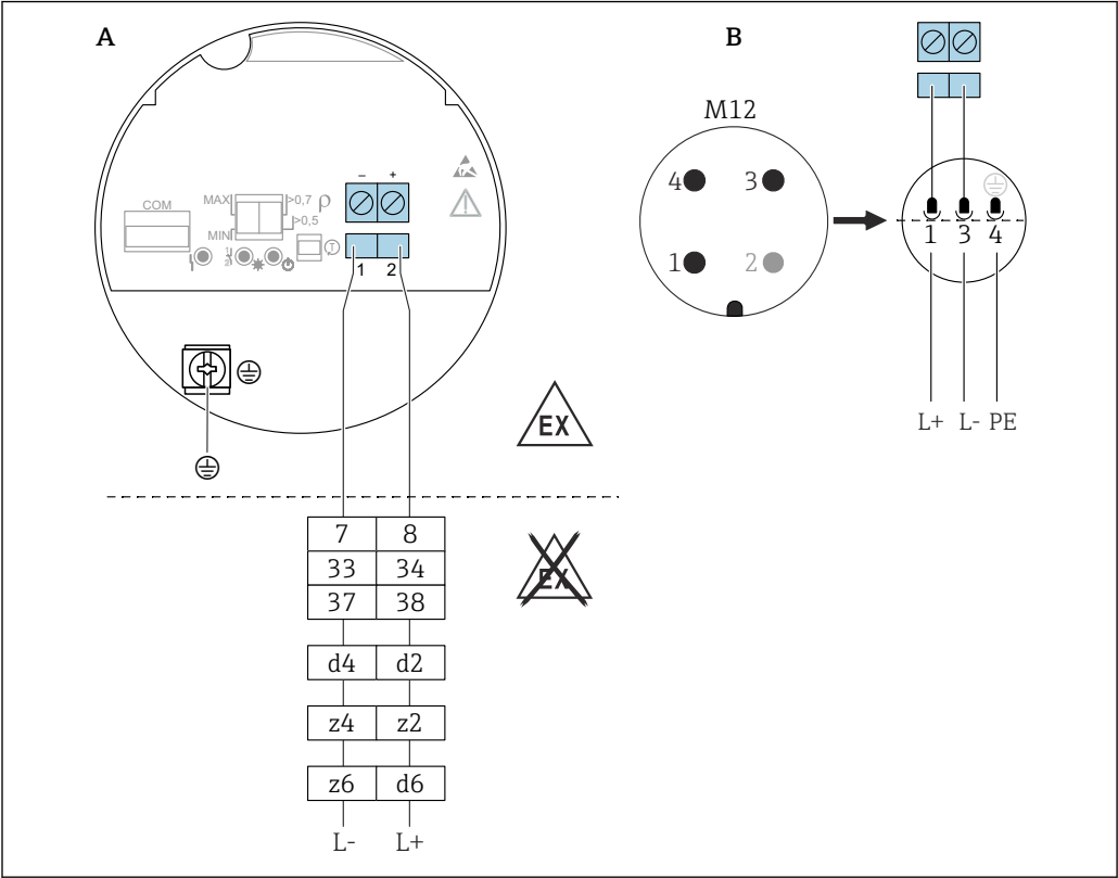
25 电子插件 FEL67: PFM 输出
