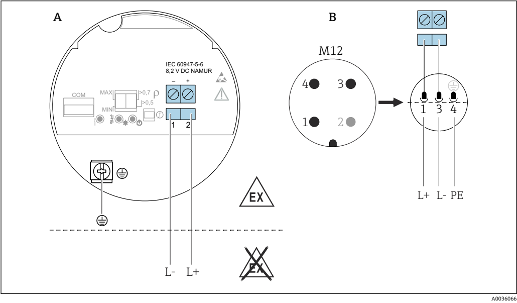
图 27 电子插件 FEL68: 两线制连接, NAMUR 信号 (≥ 2.2 mA / ≤ 1.0 mA)
