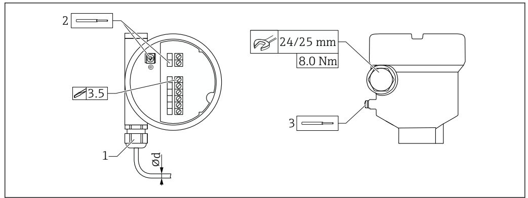
31 实例：接头（带电缆入口）和电子插件（带接线端子）
