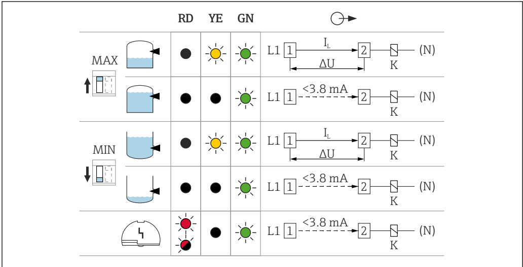
17 电子插件 FEL61 的继电器响应和故障信号
