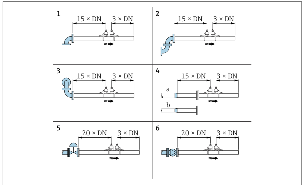
图 7 不使用 FlowDC 以及使用 1 或 2 个传感器套件以及不同节流装置时的最小前后直管段长度
