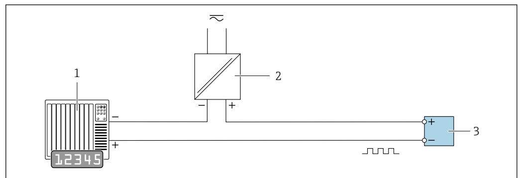
图 40 接线实例: 脉冲/频率输出 (无源信号)
