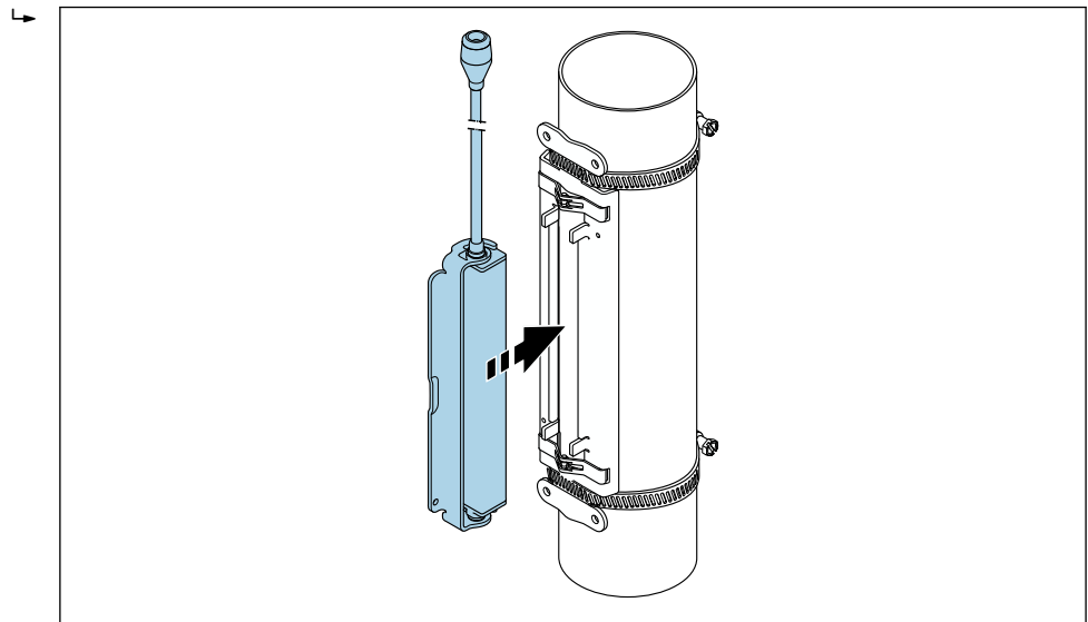
图 25 安装传感器外壳
