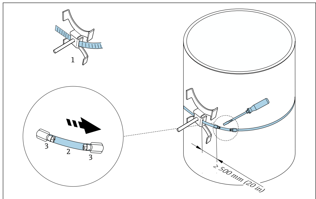
图 22 带捆扎带的传感器安装支座（大公称口径）
