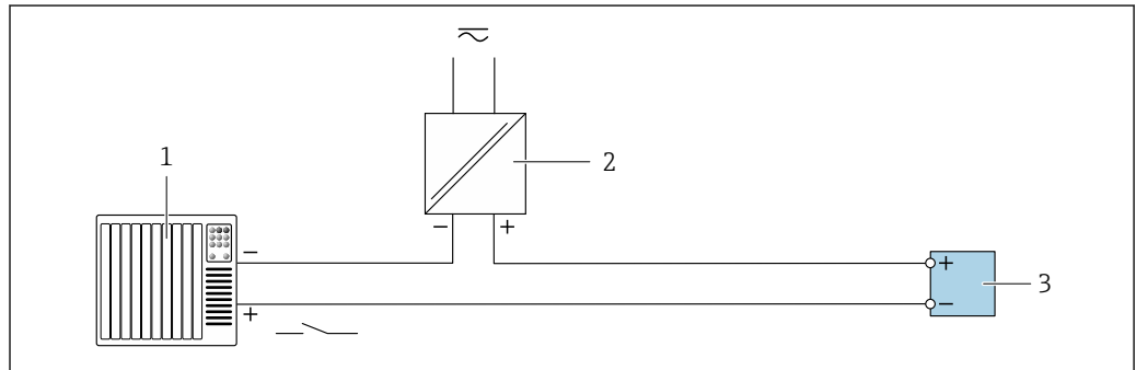
图 42 状态输入的连接实例
