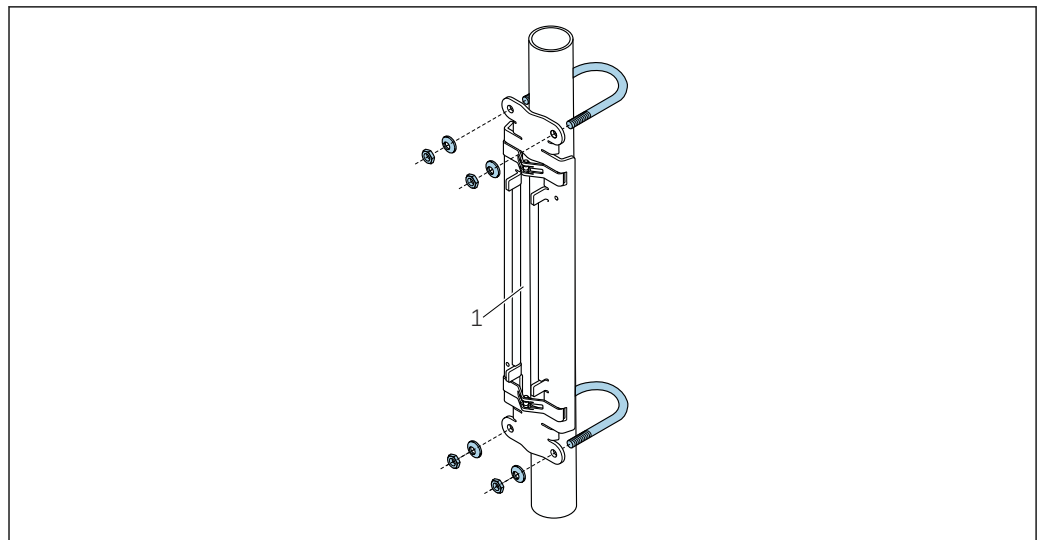
图 17 带 U 型螺丝的传感器安装支座
