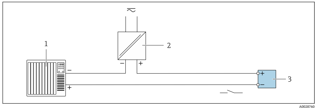
图 41 开关量输出(无源信号)的连接实例
