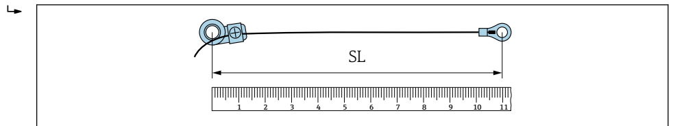
图 27 固定件与电缆接线头之间的距离等于测量线长度 (SL)
