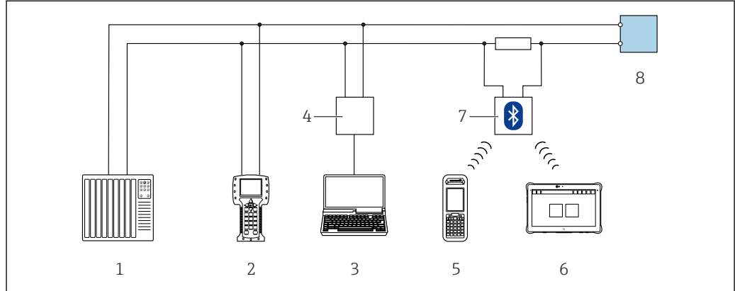
图 45 通过 HART 通信进行远程操作
