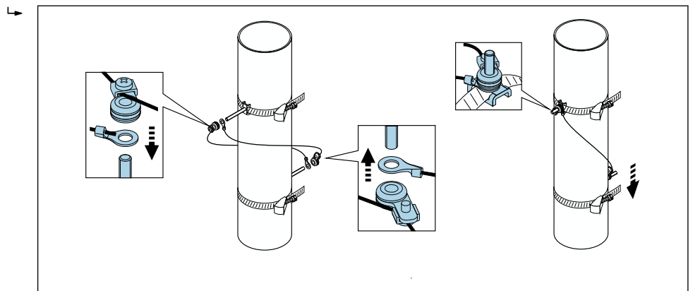
图 28 定位捆扎带 (步骤 2...4)
