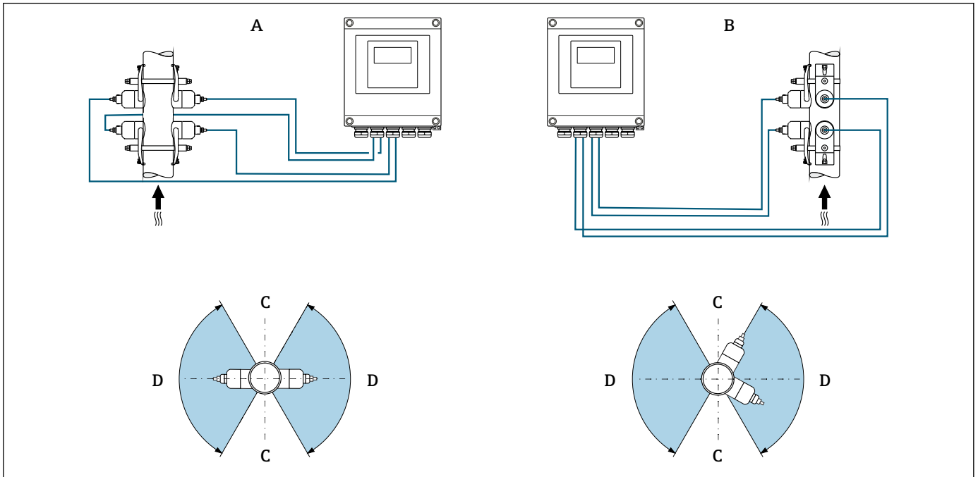
图 8 双声路测量：传感器套件在测量点处水平布置实例
