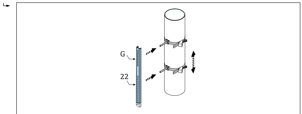
图 32 根据安装轨（例如 G22）确定距离
