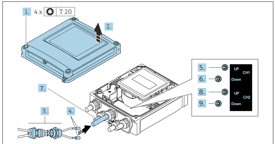
图 37 变送器：带接线端子的主要电子模块
