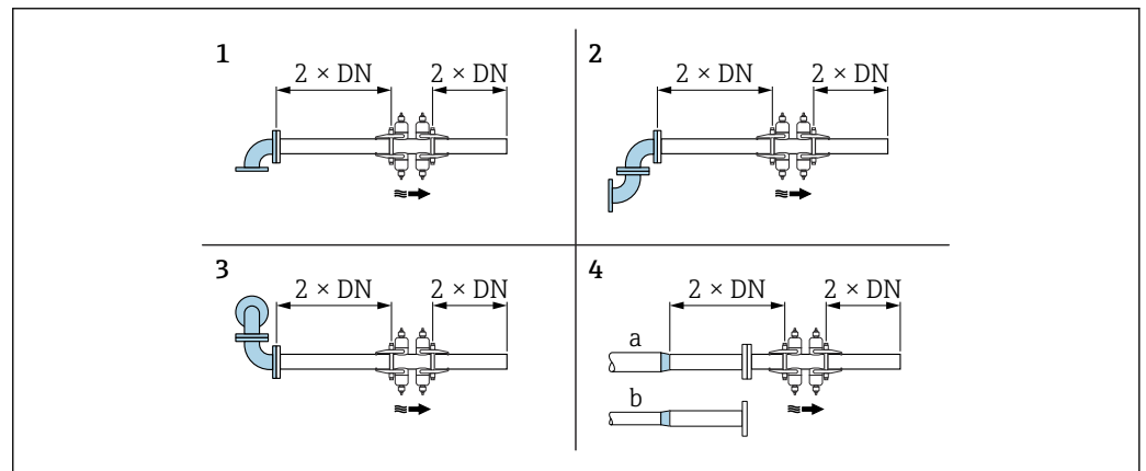
图 6 使用 FlowDC 和不同节流装置时的最小前后直管段长度
