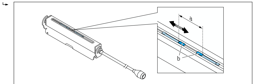
图 24 符合安装距离要求的传感器间距 → 26
