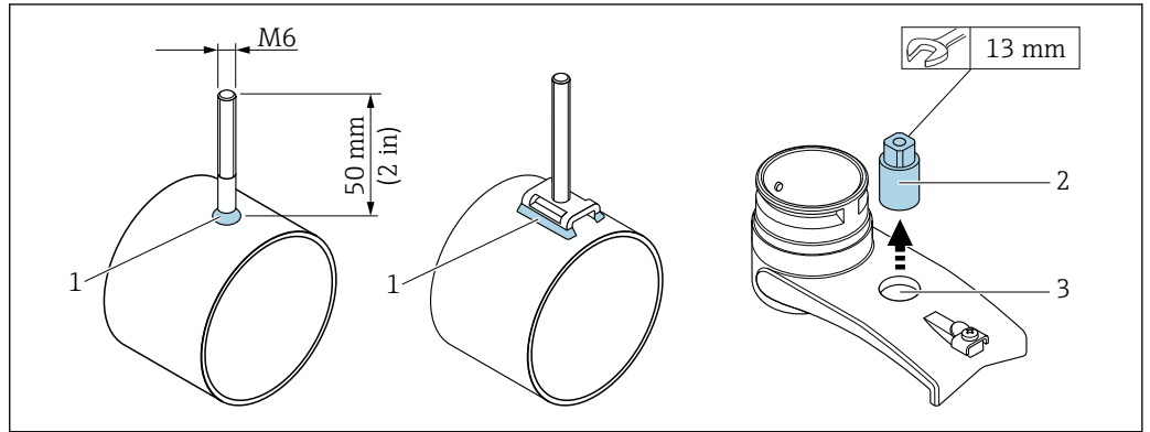
图 23 带焊接螺栓的传感器安装支座
