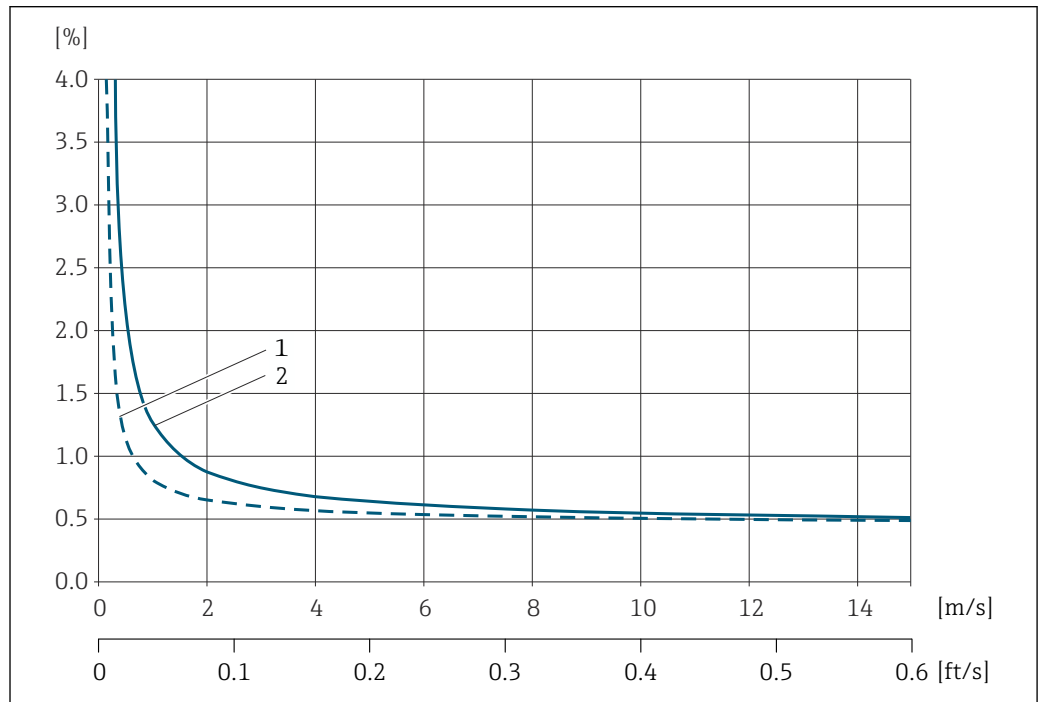
图 56 最大测量误差 (体积流量) (% o.r.) 的计算实例
