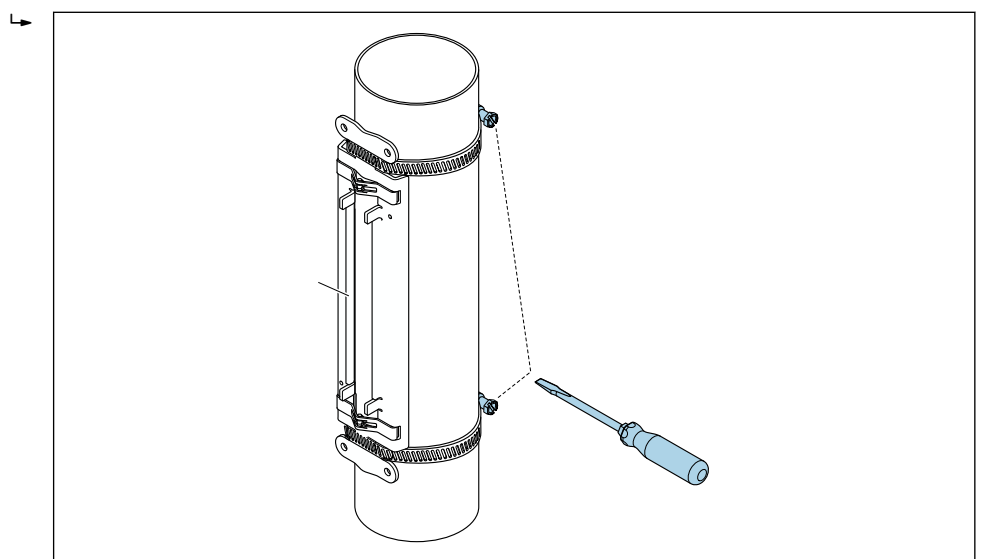
图 19 拧紧捆扎带的张紧螺丝
