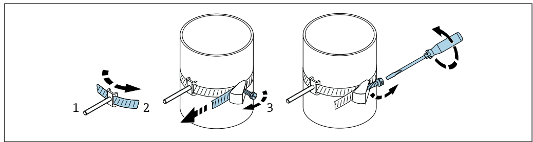
图 20 带捆扎带和铰接螺丝的传感器安装支座（中等公称口径）
