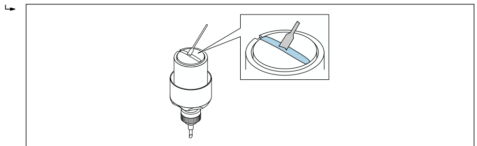
图 33 在传感器的接触面上涂抹耦合凝胶（如果没有耦合垫）
