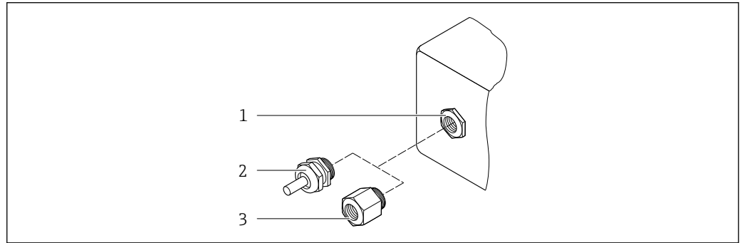
图 57 允许的电缆入口/缆塞
