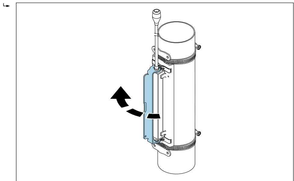
图 26 固定传感器外壳
