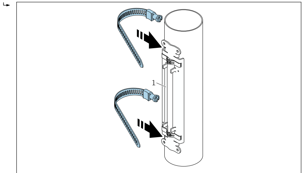
图 18 定位传感器安装支座并安装捆扎带
