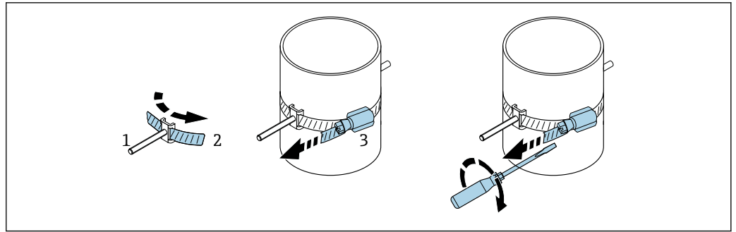
图 21 带捆扎带，不带铰接螺丝的传感器安装支座（中等公称口径）
