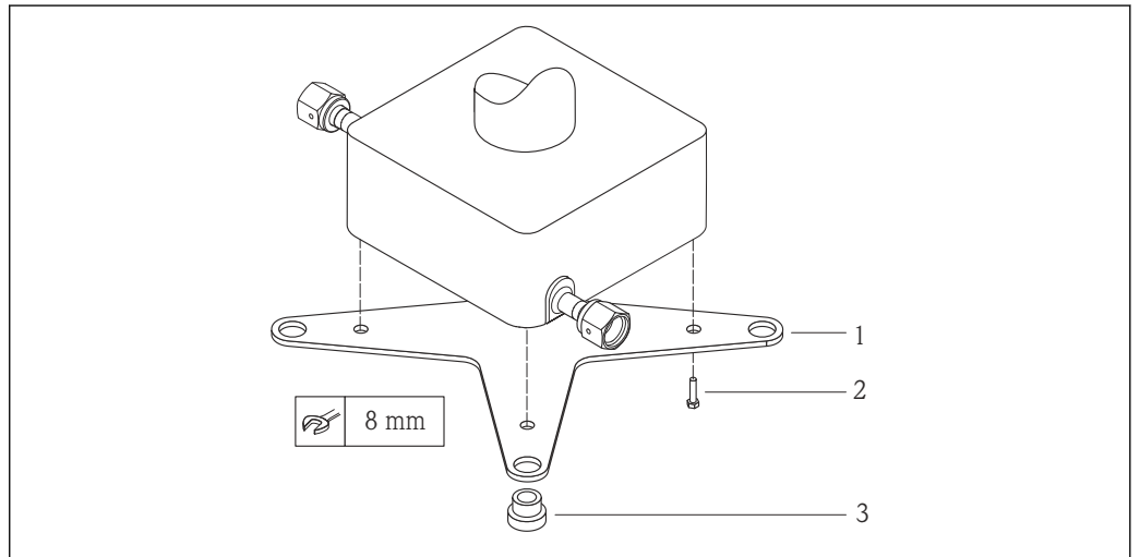
图 22 Cubemass 安装底板的安装套件示意图
