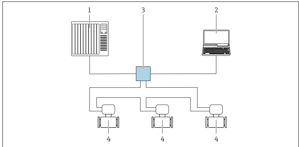
图 50 通过 PROFINET 网络实现远程操作：环形拓扑结构
