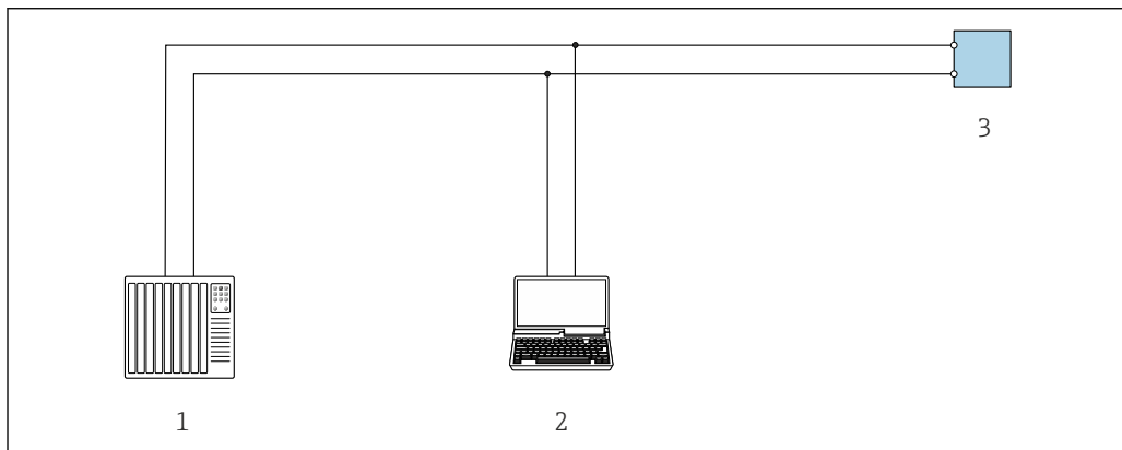
图 46 通过 Modbus-RS485 通信进行远程操作(有源信号)
