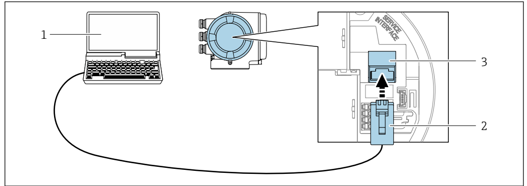
图 51 通过服务接口 (CDI-RJ45) 连接
