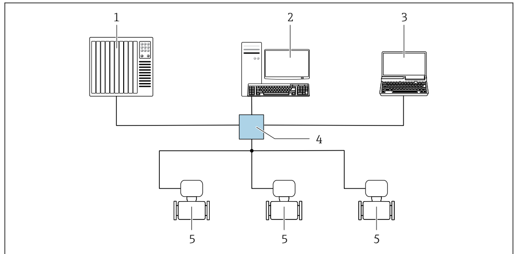
图 47 通过 EtherNet/IP 网络实现远程操作：星形拓扑结构
