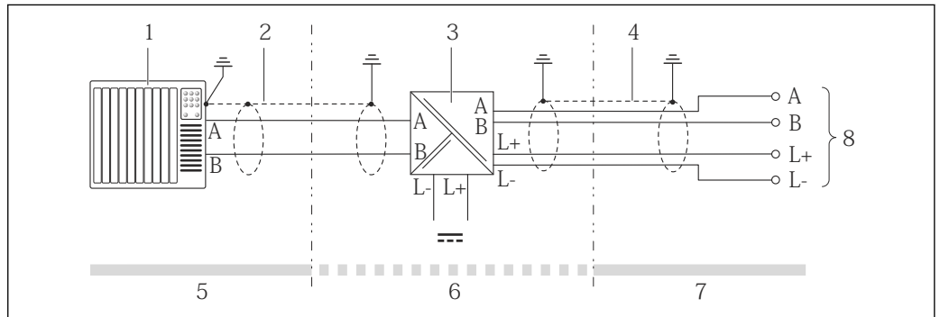
图 3 本安型 Modbus RS485 的连接示例
