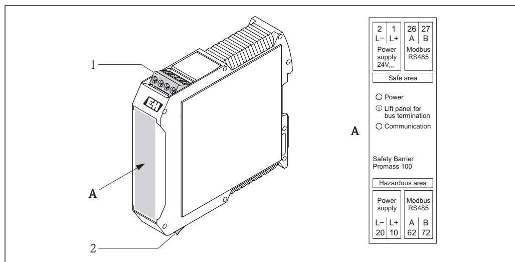
图 2 Promass 100 安全栅和接线端子示意图
