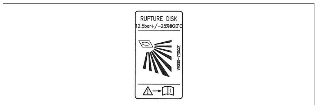
图 4 爆破片标签示意图
