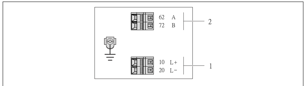
1 Modbus RS485 型仪表的接线端子分配示意图, 连接类型适用于在本安防爆场合中使用(通过 Promass 100 安全栅连接)
