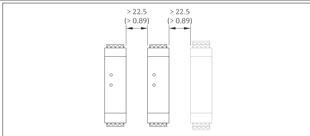
图 5 Promass100 安全栅或其他模块间的最小安装距离。单位：mm (in)
